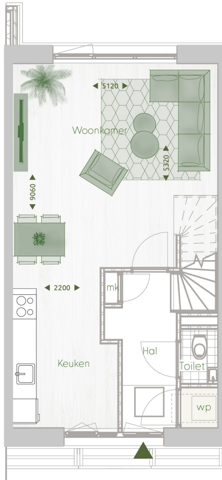
BEGANE GROND
